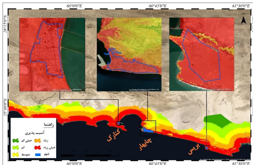
شکل ۱۶. ارزیابی آسیب پذیری خطر سونامی شهرهای استان سیستان و بلوچستان پس از بررسی آسیب پذیری شهرهای ساحلی استان سیستان و بلوچستان (شکل ۱۶) نتایج زیر حاصل گردید:
