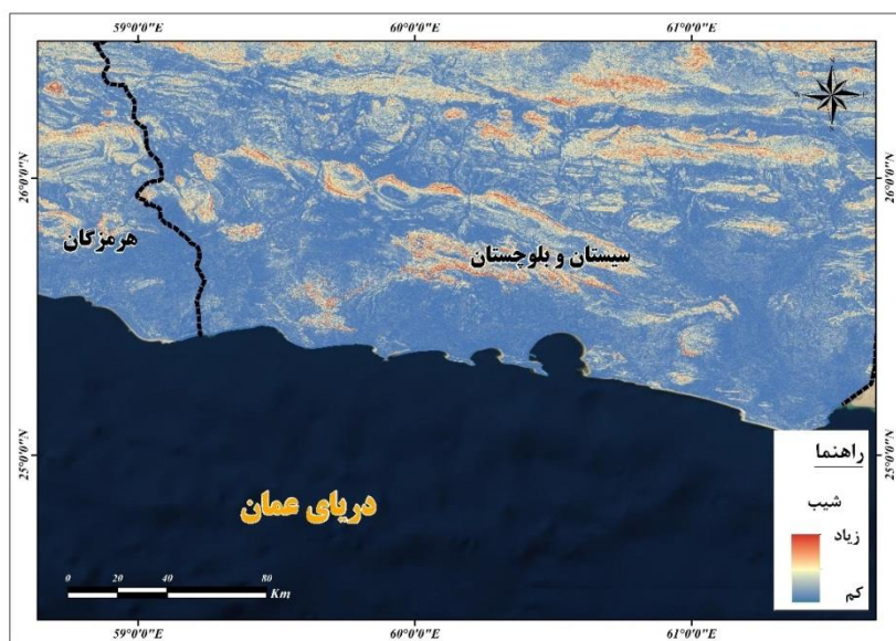
شکل ۵. شیب استان سیستان و بلوچستان
